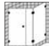
Seiteneinstieg, 1 Drehtür, 2 Festteile:
